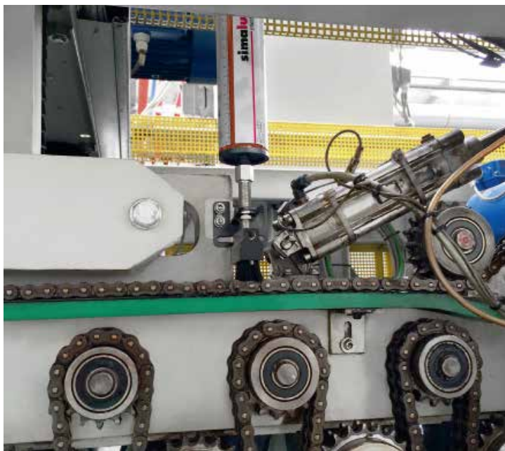
シマルーベ250により一年間チェーンへの給油が自動的に行われている例
