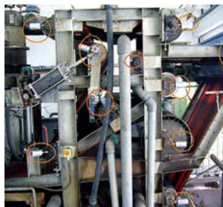
ベルトフィルタープレス機に取り付けられた無数のシマルーベ
